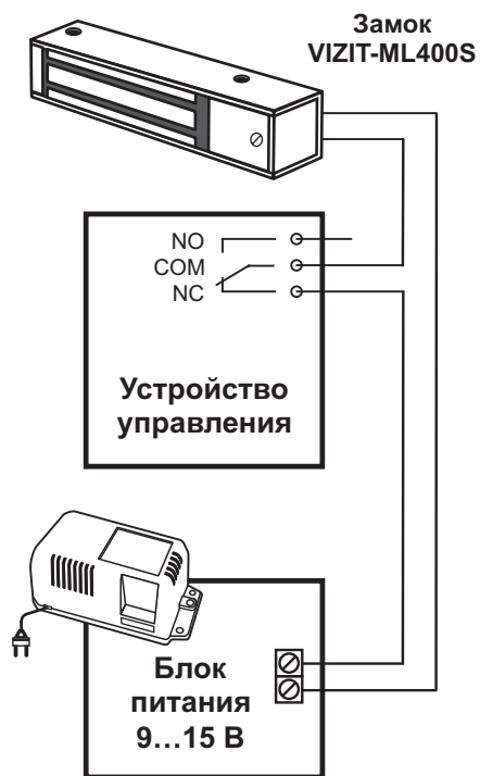
Рисунок 3 - Схема включения замка
